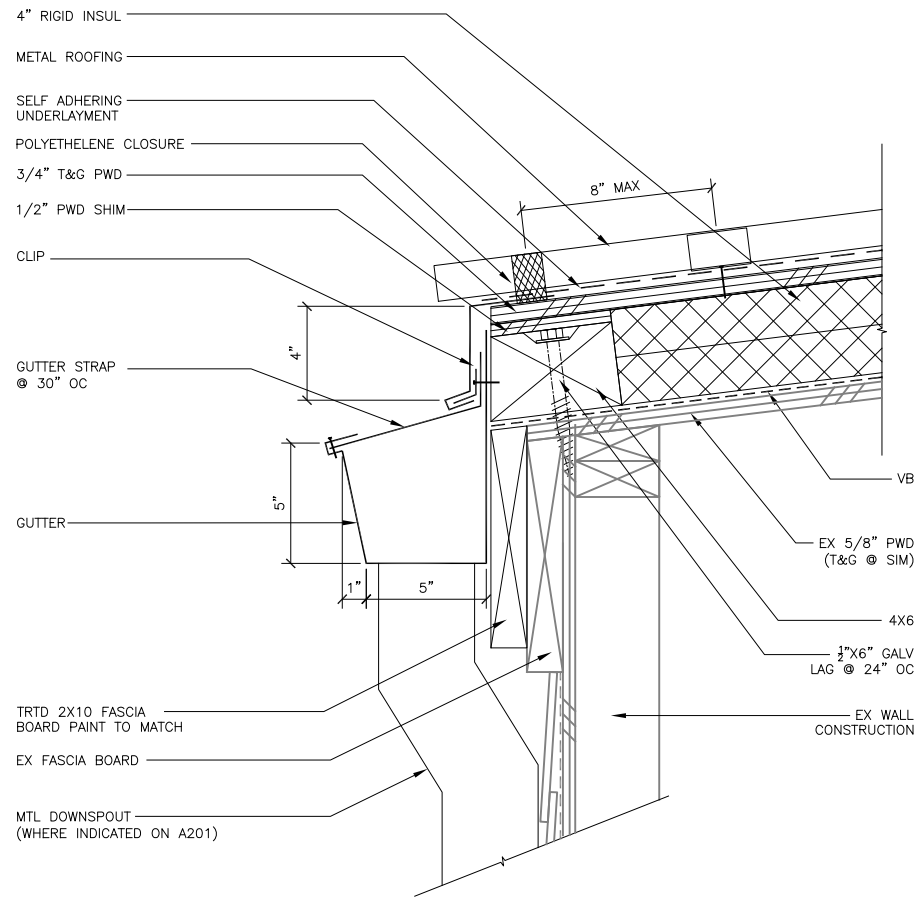
1 EAVE 11086/X_A801-1 SCALE: 0 3" 6" 1'
